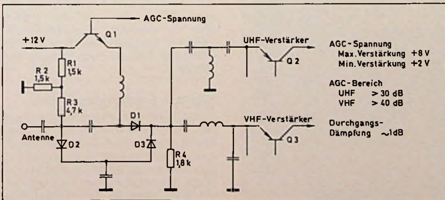
Bild 5. PIN-Dioden-Regelschaltung
