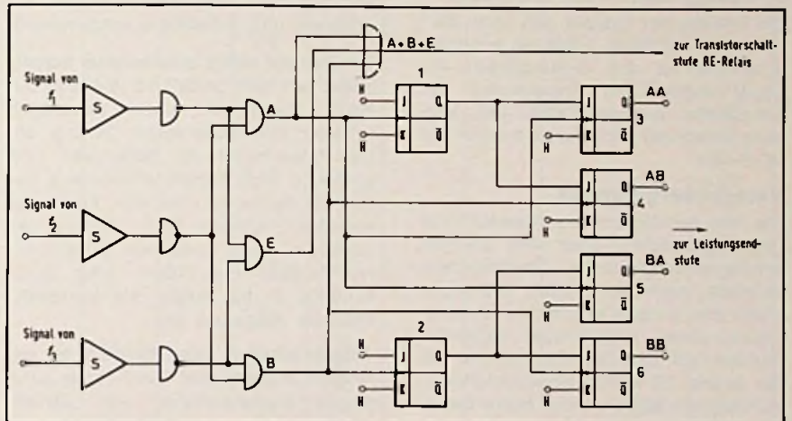
Bild 10. Auswertelogik
