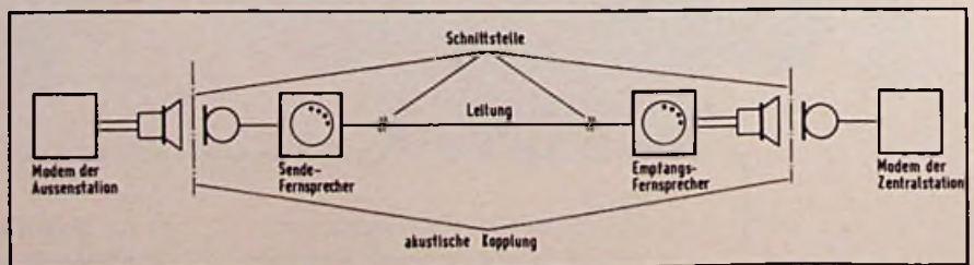
Bild 2. Blockschaltbild der Übertragungsstrecke in Senderichtung
