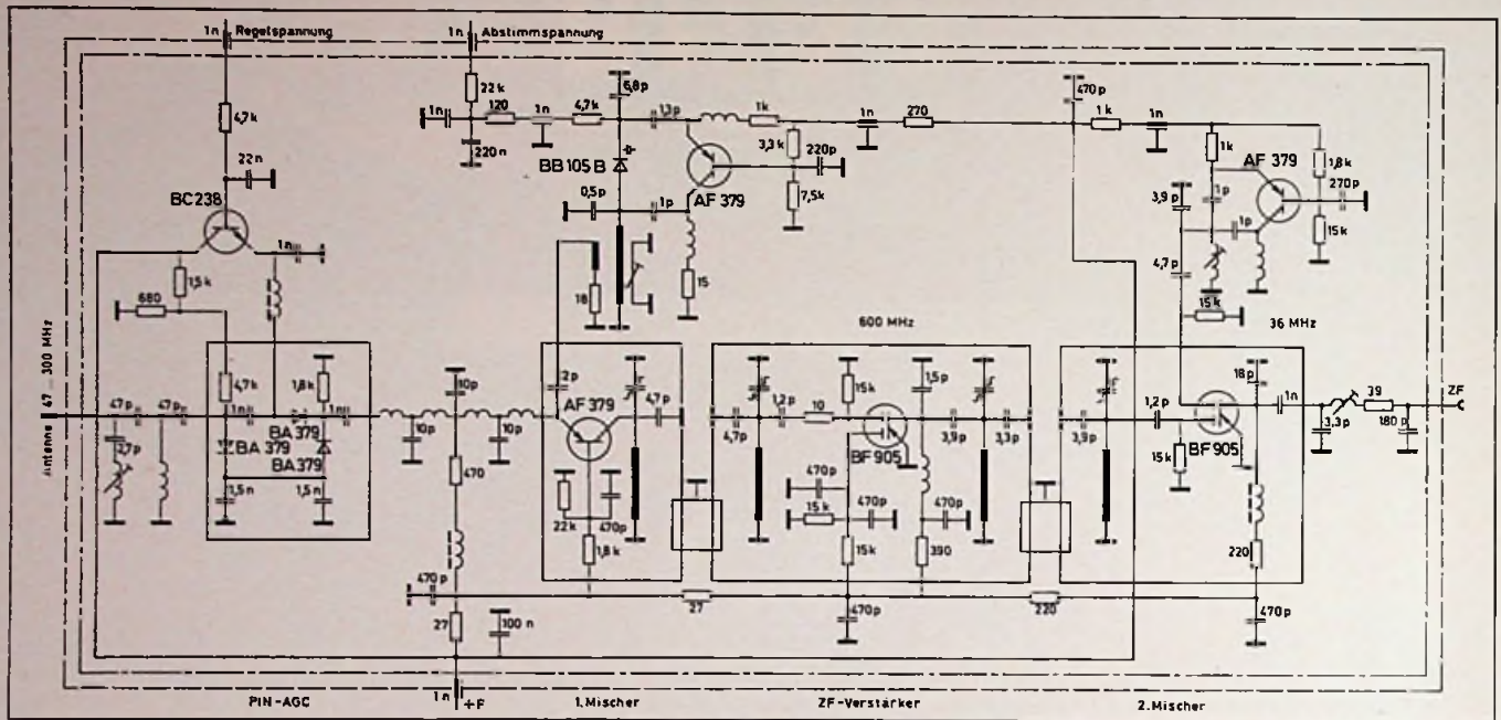
Bild 9. Schaltbild eines Kabelfernseh-Tuners mit doppelter Umsetzung
