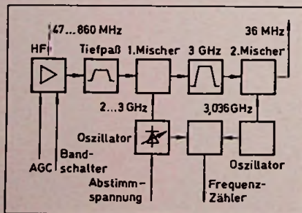
Bild 10. Blockschaubild eines UHF-VHF-Tuners mit doppelter Umsetzung und varaktorabgestimmtem Oszillator
