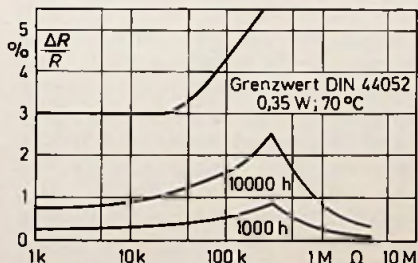
Bild 1.4. Relative Änderung bei Belastung von Kohleschichtwiderständen
