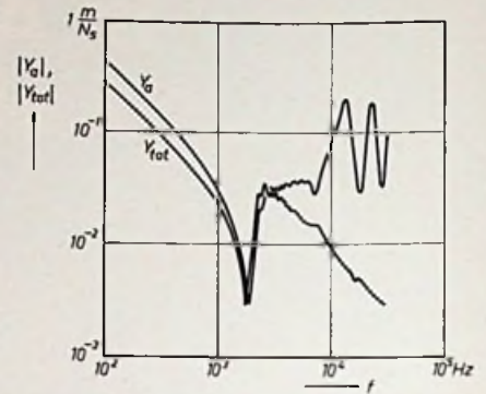
Bild 13. Berechnung der totalen axialen Admittanz Y_{tot} in Abhängigkeit von der Frequenz unter Einbeziehung der Schwingspulenmasse bei Konus 50.1. Zum Vergleich ist die Kurve Y_a von Bild 12 noch einmal eingezeichnet.
