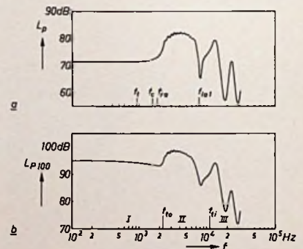
Bild 14. a) Schalldruckpegel L_p auf der Achse von Konus 50.1 (errechnete Kurve unter Vernachlässigung der Schwingspulenmasse; Entfernung 10 m, Antriebskraft 1 N). Der Pegel ist in Dezibel ausgedrückt, bezogen auf 20 \mu Pa . b) Der Pegel L_{P100} der Schalleistung, die in einem Kegel mit einem Spitzenwinkel von 100^\circ abgestrahlt wird. Der Pegel L_{P100} ist in Dezibel ausgedrückt, bezogen auf 10^{-12} W . Eine Anzahl charakteristischer Frequenzen sowie die Frequenzbereiche I, II und III sind angegeben.
