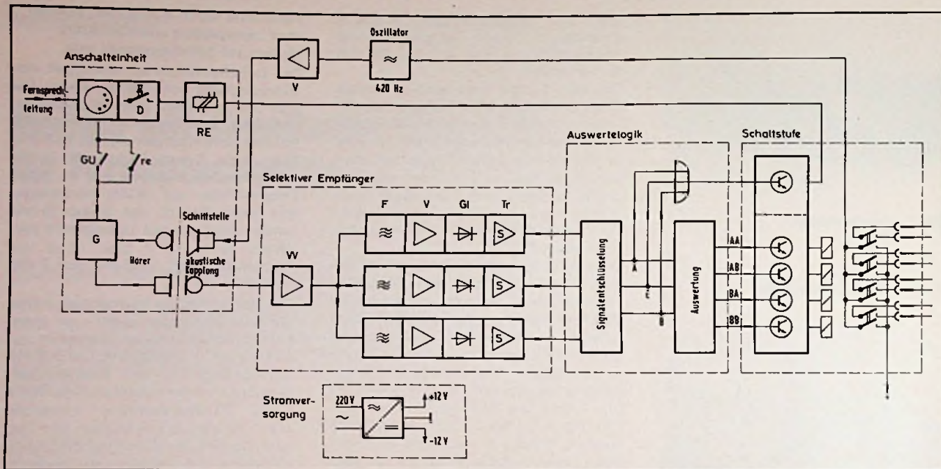
Bild 7. Blockschaltbild des Empfängermodems; es bedeuten: D Datentaste, RE Rufempfangsrelais, GU Gabelumschalter, G Gabel, VV Vorverstärker, F aktives Filter, V Zwischenverstärker, Gl Gleichrichtung und Verzögerung, Tr Trigger, A Signalkombination aus f_1 und f_2 , B Signalkombination aus f_2 und f_3 , E Ruhekombination aus f_1 und f_3
