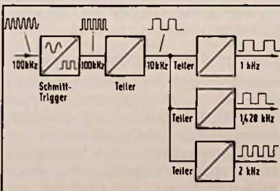
Bild 5. Blockschaltbild des Frequenzteilers im Modem der Außenstation
