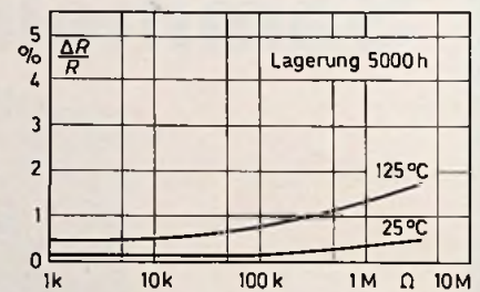
Bild 1.3. Relative Änderung bei Lagerung von Kohleschichtwiderständen
